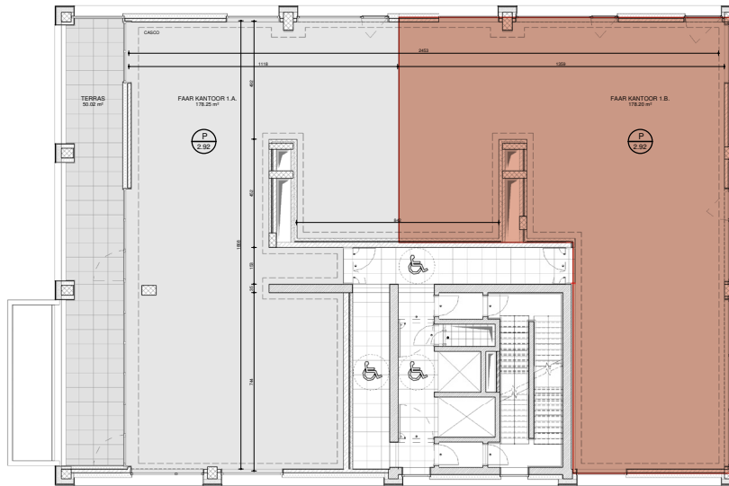
Verdieping +01
