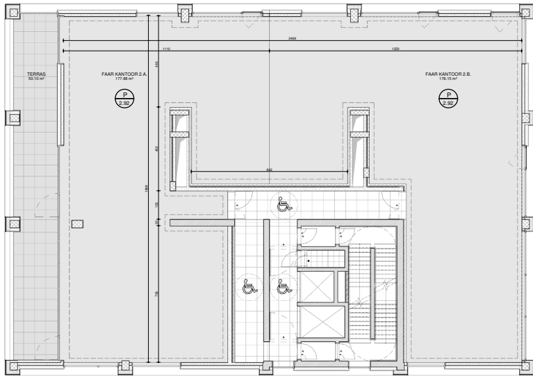
Verdieping +02
